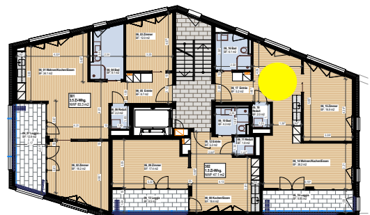
Grundriss 3. OG Haus 2a „Ahorn“
